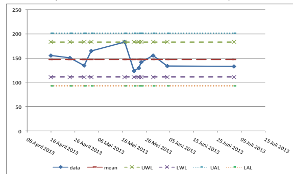
Gambar 3d Pengecekan untuk tegangan 120 V, arus 5 A, frekuensi 53 Hz dan PF = 0,5 lag.
